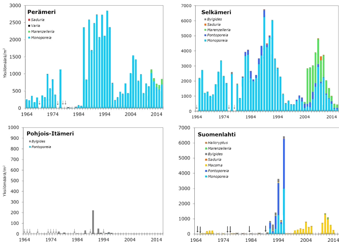
Kuva 53. Pohjaeläimistön yhteisörakenteen pitkäaikaismuutokset seurantaohjelman havaintopaikoilla avomerellä. Nuolet osoittavat vuodet jolloin havaintopaikalla ei ole otettu näytteitä. Lajinimet: Saduria entomon: kilkki, Monoporeia affinis : valkokatka, Pontoporeia femorata : merivaikkatka, Bylgides sarsi : liejusukasjalkainen, Halicryptus spinulosus : okamakaramato, Marenzelleria sp.: liejuputkimato, Macoma balthica (nyk. Limecola balthica ): liejusimpukka, varia: muut satunnaiset lajit. Huomaa y-akselin erilaiset asteikot.
